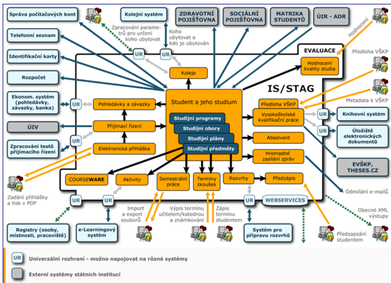
Schema IS/STAG a jeho napojení na další systémy
