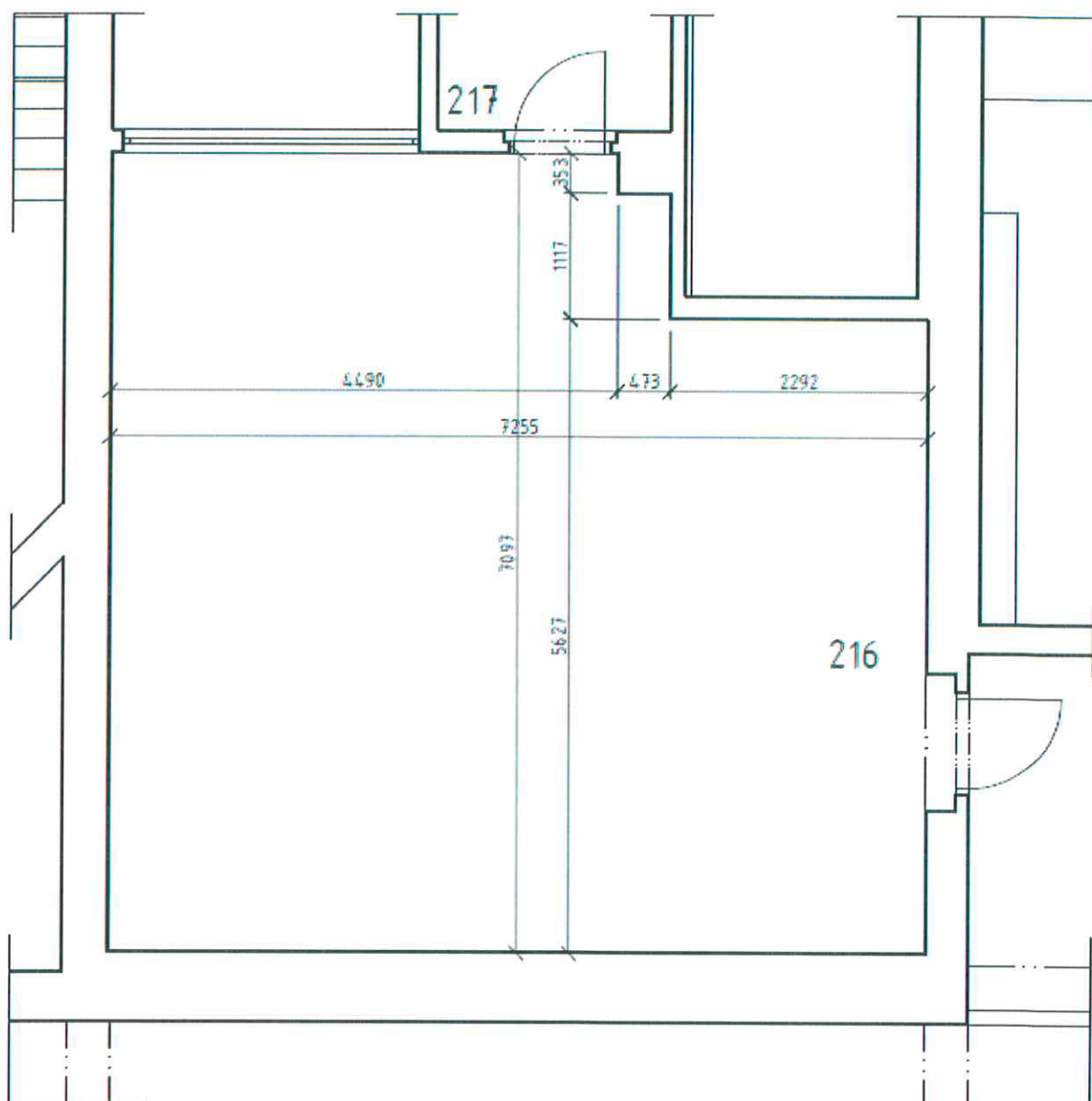
Obrázek 1 Půdorys místnosti UV216
