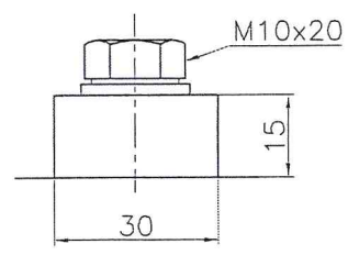
DETAIL ZEMNÍCÍ SVORKY
