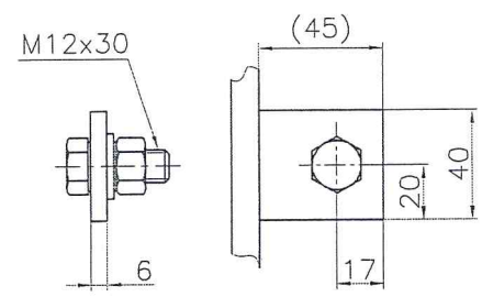
DETAIL PŘIPOJOVACÍ SVORKY
