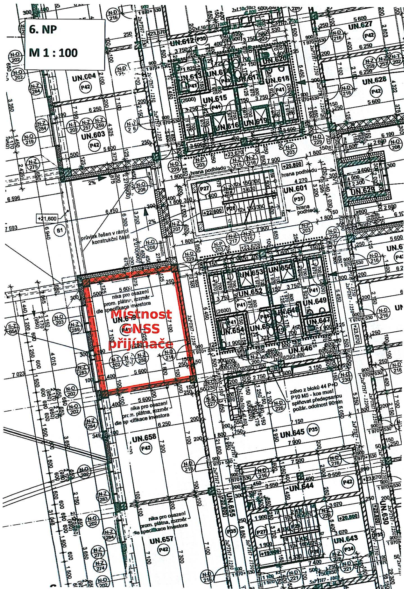
Příloha č. 3: Výkresová dokumentace stavební připravenosti místa instalace Zařízení
